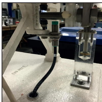
Nieuw voorweegsysteem
